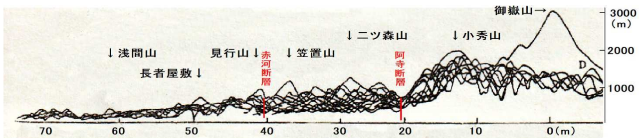
図3 美濃・阿寺山地の投影断面図（木曾敏行、1963より引用・加筆）
