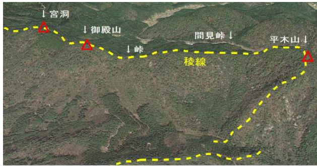
図 52 稜線の連続 (Google Earth で作成加筆) 南方からの鳥瞰画像
