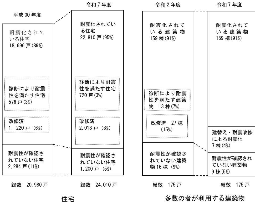
図 2 - 4 住宅・多数の者が利用する建築物の耐震化の目標(令和 7 年度)
